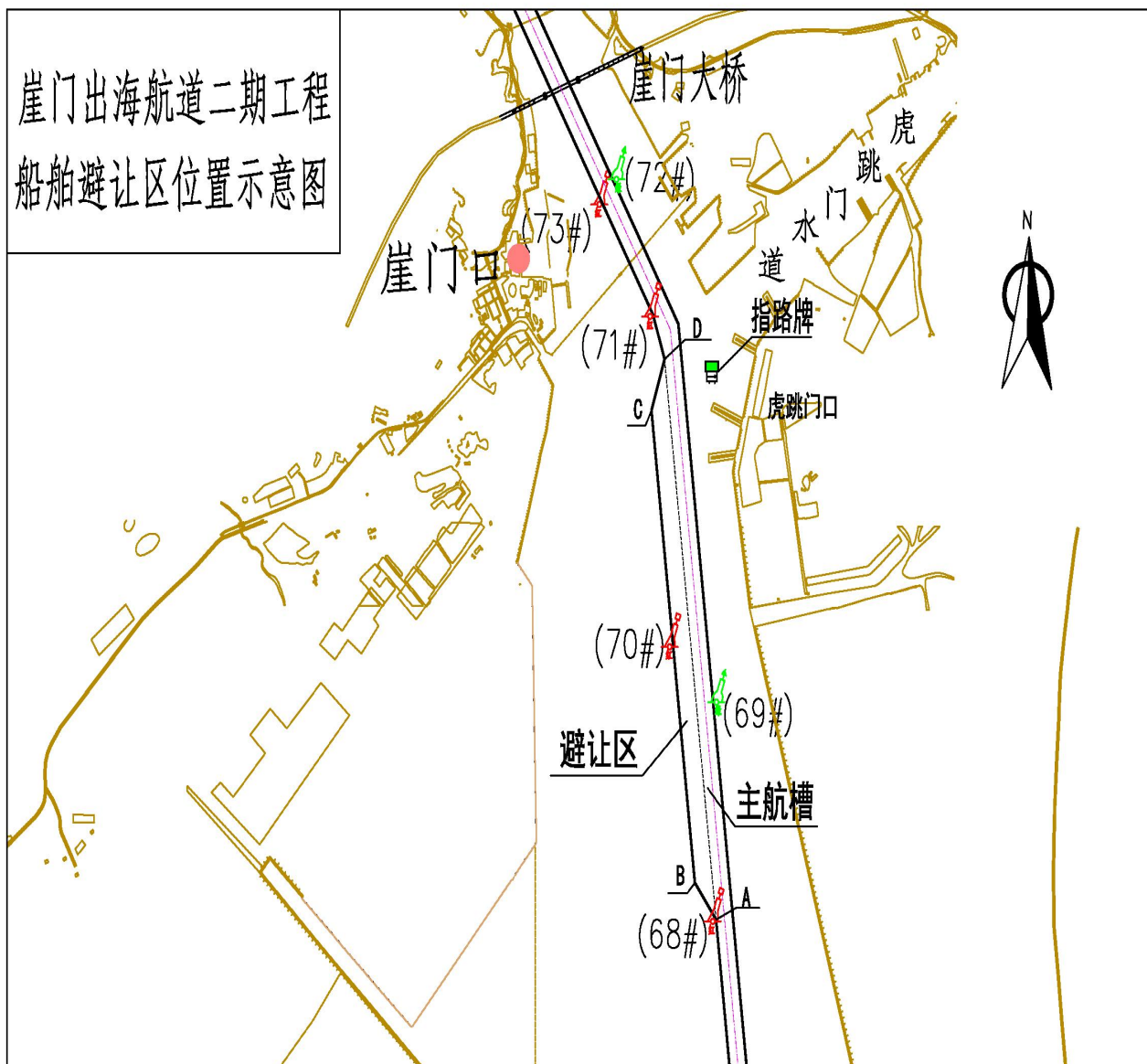
崖门出海航道二期工程船舶避让区位置示意图
