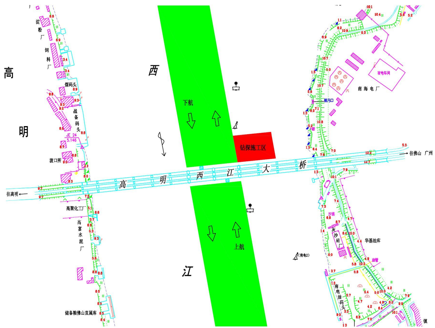
西江高明大桥上游清礁工程地质勘察第二阶段通航方案及航标配布示意图
