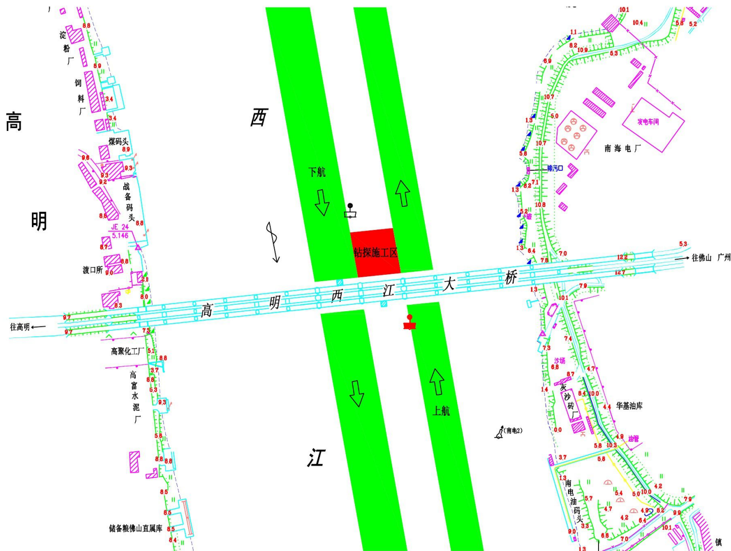
西江高明大桥上游清礁工程地质勘察第一阶段通航方案及航标配布示意图 (白天)
